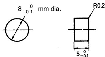
V600-D23P53
