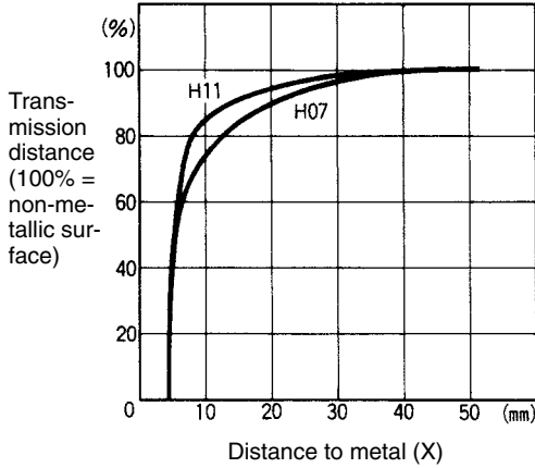
(1) V600-D23P71
