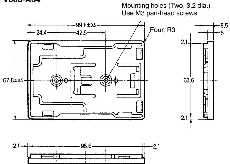
V600-A84
