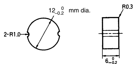
V600-D23P54
